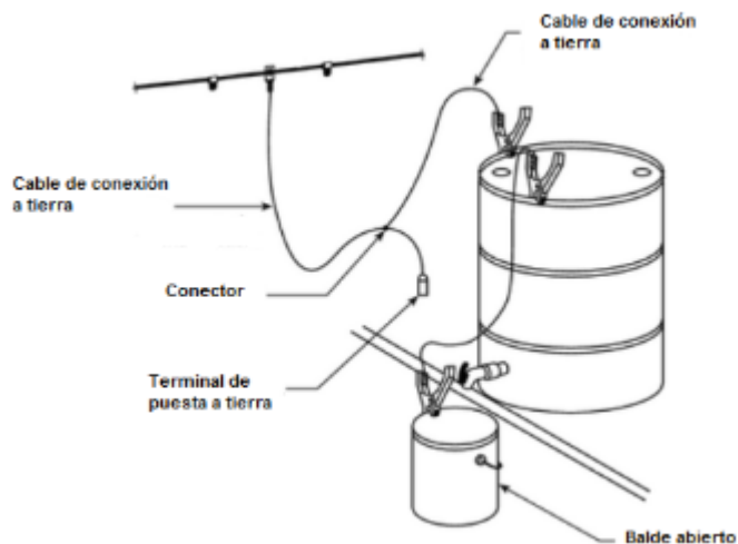
c) Sistema a tierra típico para despacho de solvente de bajo volumen vía conector de tambor.
