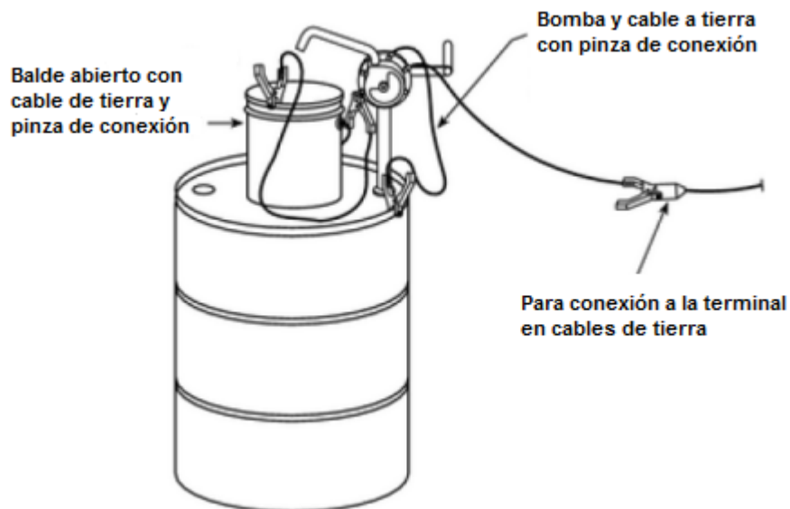
d) Sistema a tierra típico para despacho de solvente de bajo volumen vía bomba de tambor.
